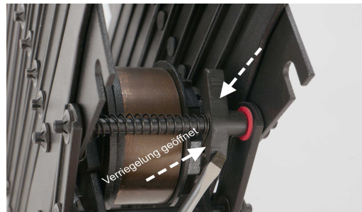
Bild: Verriegelung geöffnet
